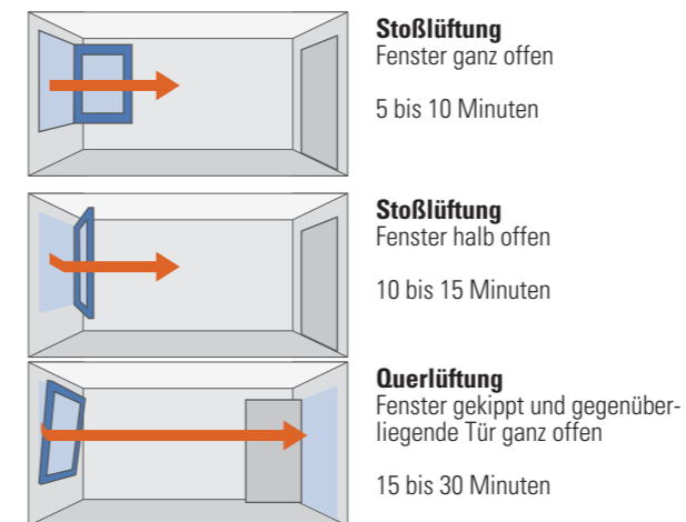
Durchschnittliche Dauer des Luftaustauschs je nach Fensterstellung
