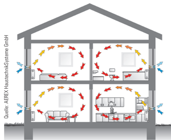
Dezentrale Lüftungsanlage
