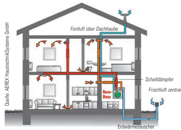
Zu- und Abluftanlage mit Wärmerückgewinnung
