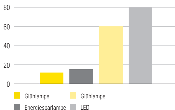
Lichtausbeute (lm/W)
